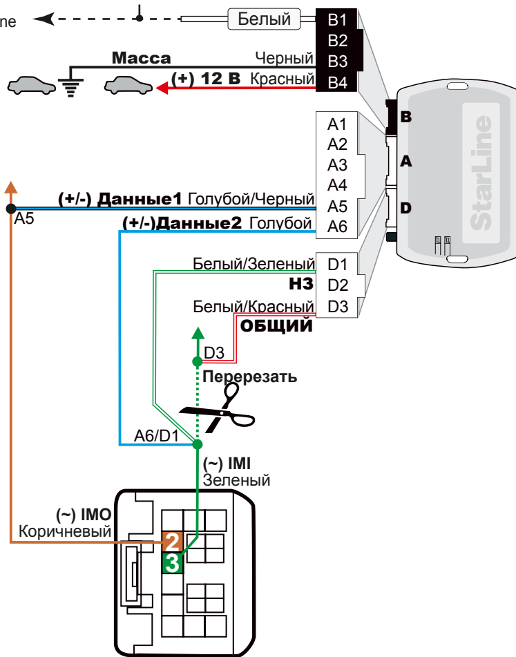
Белый 18-контактный разъем. Вид сзади.
